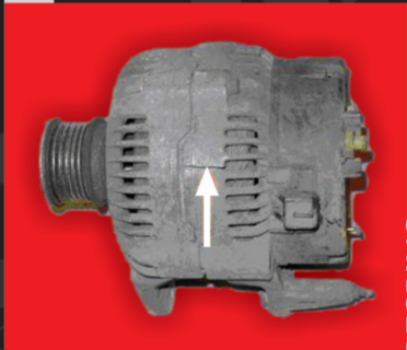
2. Carcasă fisurată
